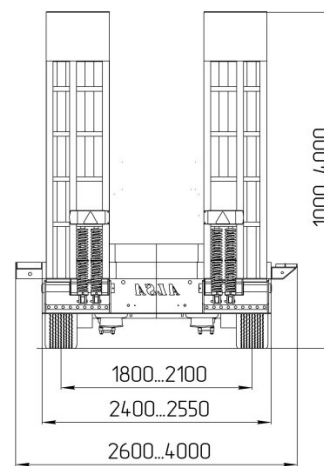
Вариант исполнения с двухступенчатыми трапами
