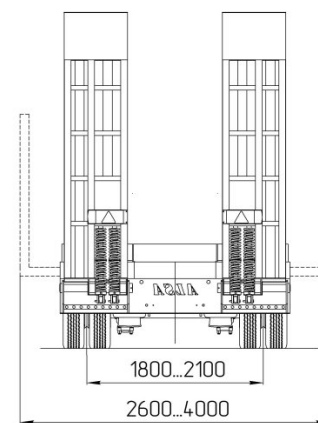
Вариант исполнения с гидравлическими трапами
